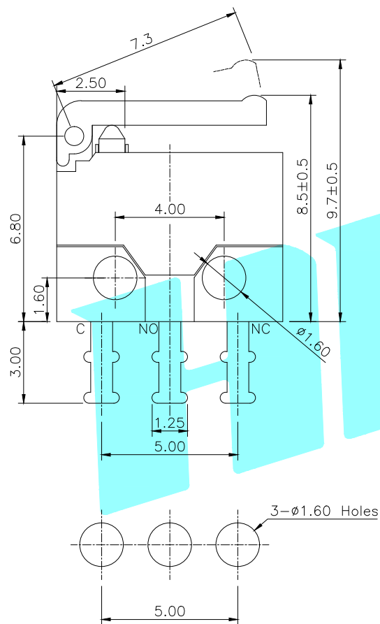
PCB Layout(Pattern side)
